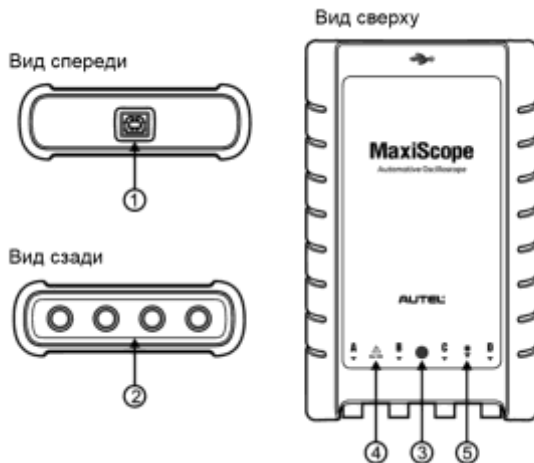
Рисунок 15-3 Вид осциллографа спереди, сзади и сверху
