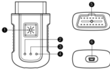
Рисунок 2-4 Беспроводной диагностический интерфейс MaxiVCi V100
